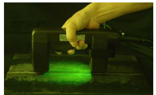
LEDブラックライト(別売) と組み合わせた使用例
