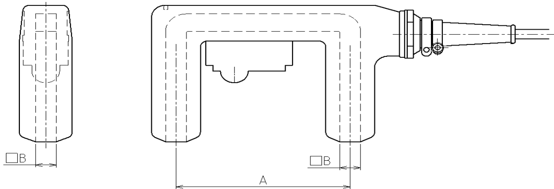
ハンドマグナの形状 (ヨーク未装着)
